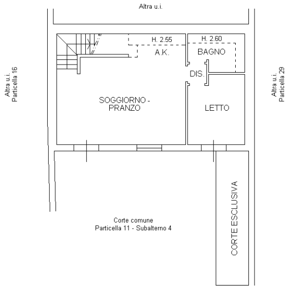
PIANO TERRA H. 2.80
