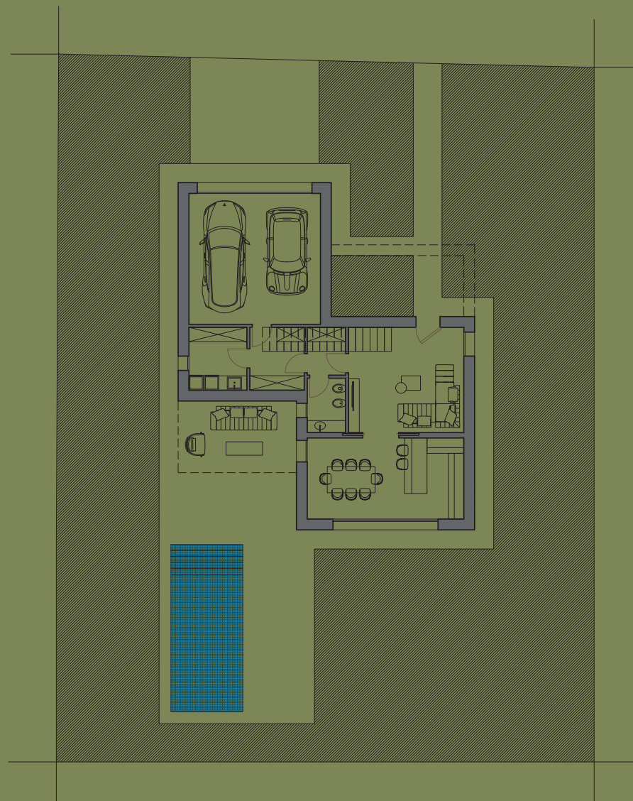
Planimetria
